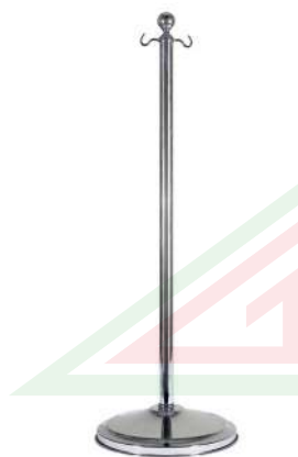
Piantana ottone cromato Ø 300 mm, fusto Ø 30 mm Ø 300 mm chrome brass column, Ø 30 mm shaft
